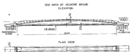
Arche d'essai du Pont du Veurdre
